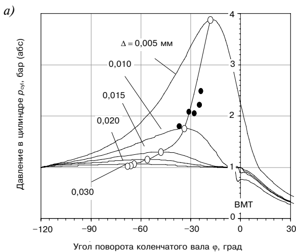
Рис. Иллюстрация изменения давления в цилиндре при проворачивании коленчатого вала валоповоротным устройством (а) и процедура поиска дискриминантной функции для диагностирования неисправности «нарушение герметичности КС» (б)
