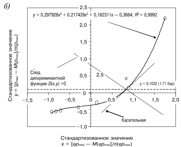
Рис. Иллюстрация изменения давления в цилиндре при проворачивании коленчатого вала валоповоротным устройством (а) и процедура поиска дискриминантной функции для диагностирования неисправности «нарушение герметичности КС» (б)
